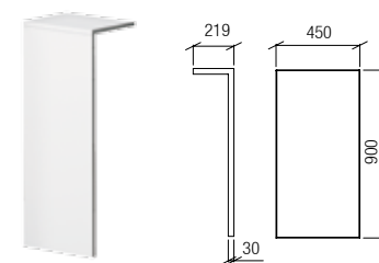
01 Vorsatzblende aus weiß beschichtetem Holzwerkstoff, mit umlaufendem Profil, aus schwarz pulverbeschichtetem Stahl
